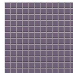
Pirrotina
