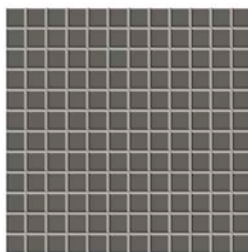
Ematite
