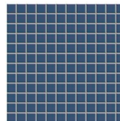
Azzurrite
