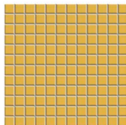
Siderite
