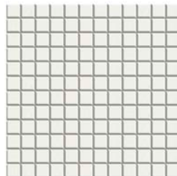
Calcite
